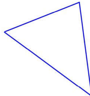
le triangle quelconque
